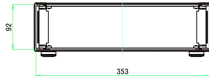
A-A ( 1 : 4.5 )
