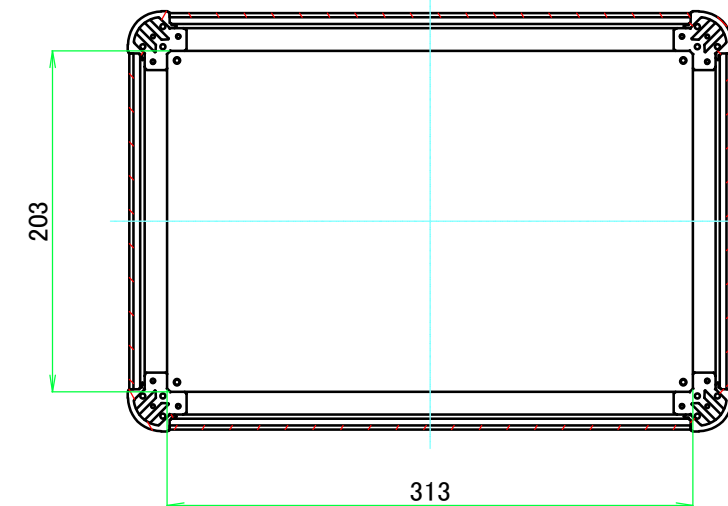
C-C ( 1 : 4.5 )
